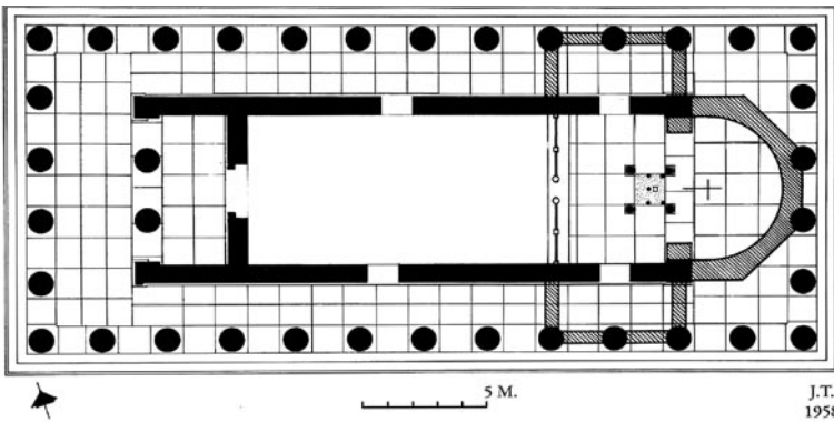
13. Κάτοψη του Ηφαισείου, όπου διακρίνεται και η μετατροπή του σε χριστιανική εκκλησία (Άγιος Γεώργιος), 7ος αι. μ.Χ.
