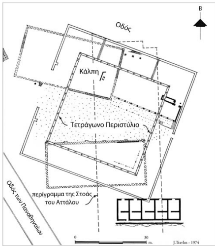
50. Κάτοψη των Δικαστηρίων κάτω από το βόρειο άκρο της Στοάς του Αττάλου, 5ος-4ος αι. π.Χ.
