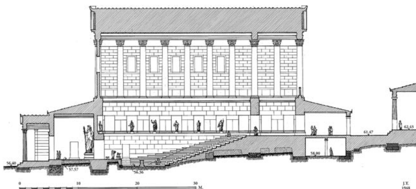
52. Τομή του Ωδείου του Αγρίππα, α' φάση (τέλη 1ου αι. π.Χ.). Άποψη από τα δυτικά.
