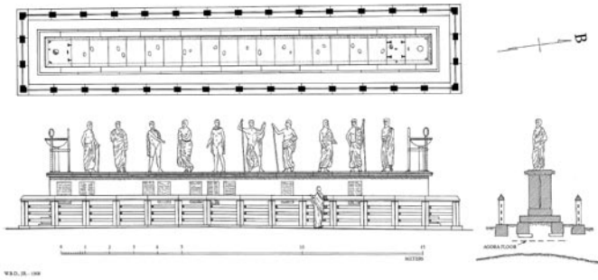
22. Αναπαράσταση του Μνημείου των Επώνυμων Ηρώων, β' μισό 4ου αι. π.Χ. Κάτοψη, όψη και τομή.
