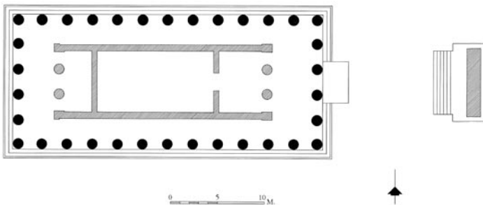
56. Κάτοψη του ναού του Άρεως (β' μισό 5ου αι. π.Χ.) που μεταφέρθηκε στην Αγορά στα τέλη του 1ου αι. π.Χ.
