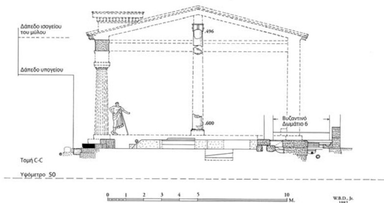
65. Τομή της Ποικίλης Στοάς, με δωρικούς κίονες εξωτερικά και ιωνικούς εσωτερικά, περ. 470-460 π.Χ.
