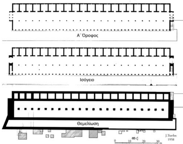
47. Κατόψεις της Στοάς του Αττάλου, 159-138 π.Χ.
