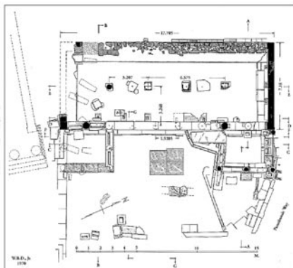
61. Σχεδιαστική αποτύπωση των λειψάνων της Βασιλείου Στοάς.
