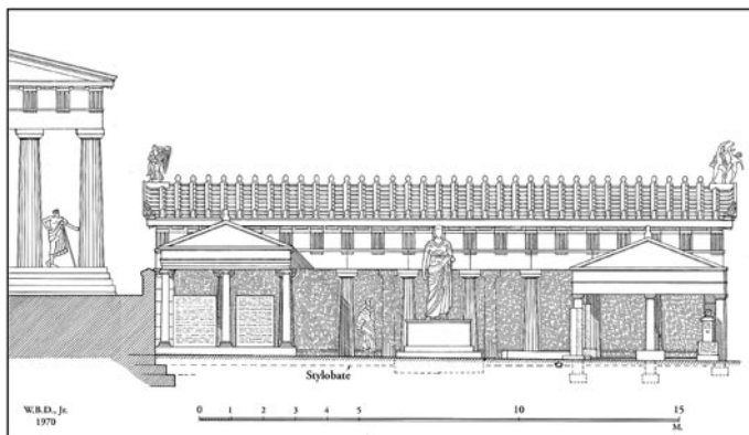
62. Αναπαράσταση της Βασιλείου Στοάς στη μορφή που είχε γύρω στο 300 π.Χ.
