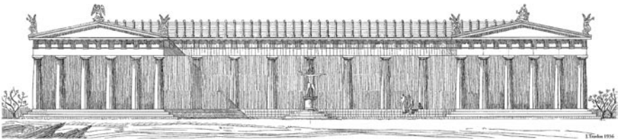
9. Αναπαράσταση της δωρικής Στοάς του Διός Ελευθερίου, περ. 430-420 π.Χ.
