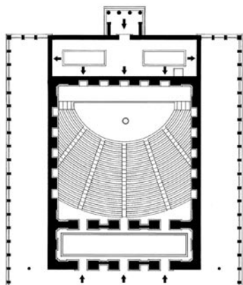
53. Κάτοψη του Ωδείου του Αγρίππα, α' φάση (τέλη 1ου αι. π.Χ.).
