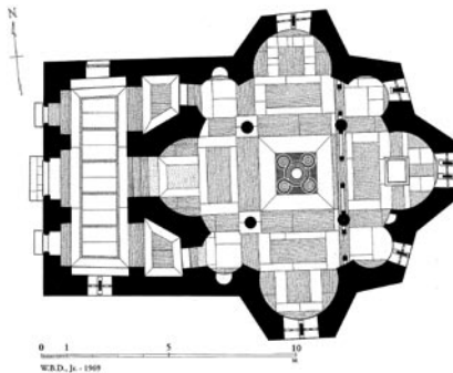
68. Κάτοψη της εκκλησίας των Αγίων Αποστόλων.
