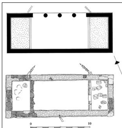
33. Αποκατάσταση της κάτοψης της Νοτιοανατολικής Κρήνης (β' μισό του αι. π.Χ.) και η σημερινή της μορφή.
