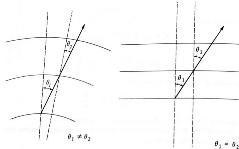
Σχήμα από Novotny Introduction to Stellar Atmospheres and Interiors
