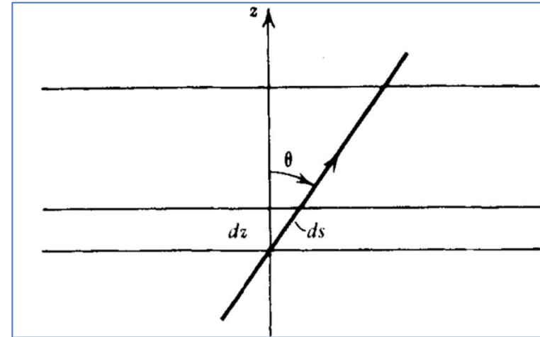
Σχήμα από Rybicky & Lightman
