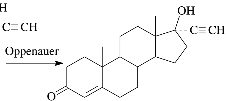
ethisterone
