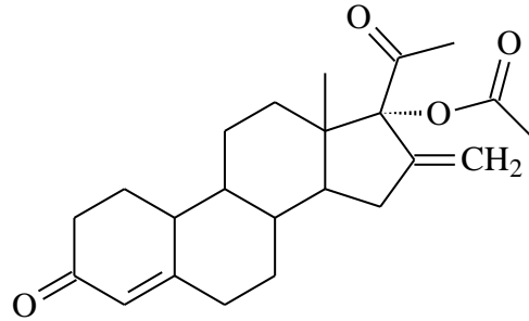
elcometrine
