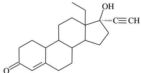
norgestrel
