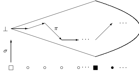
ΔΙΑΓΡΑΜΜΑ 7.3. Υπερπεπερασμένη τροχιά επεκτατικής απεικόνισης.
