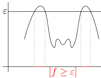
Σχήμα 7.1: Απόδειξη της ανισότητας Chebyshev-Markov
