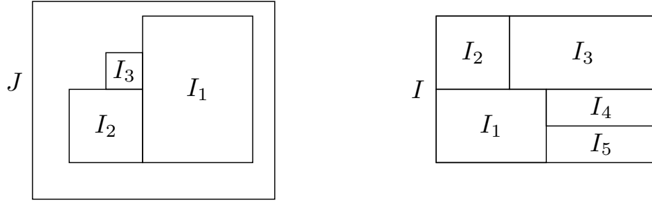
Σχήμα 3.1: Λήμμα 3.1.6 (ii)
