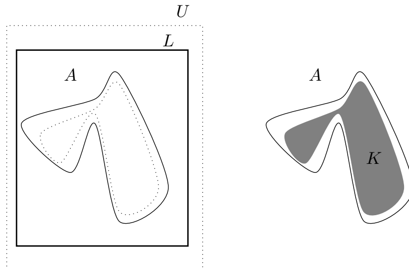
Σχήμα 4.1: Απόδειξη της εσωτερικής κανονικότητας για φραγμένα σύνολα
