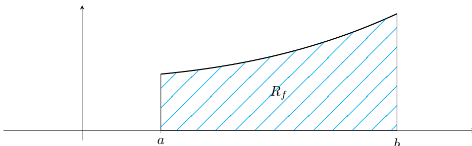
Σχήμα 1: Γεωμετρική ερμηνεία του ολοκληρώματος
