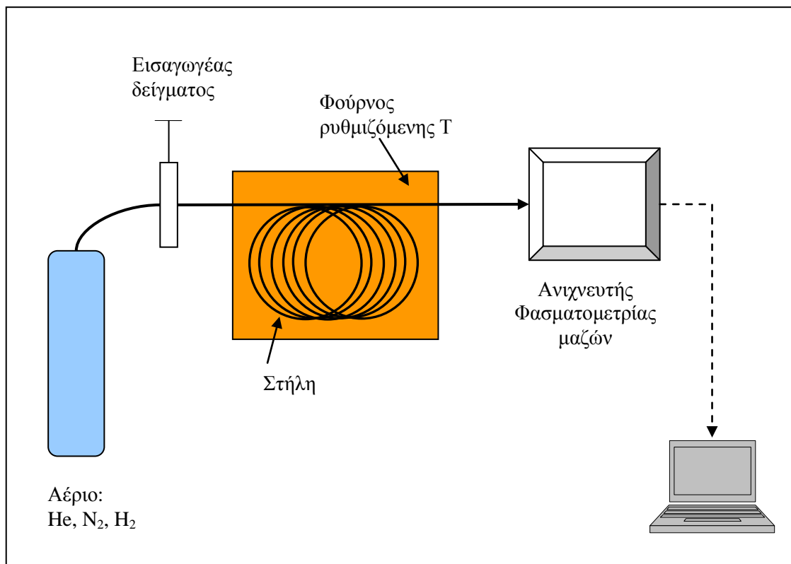
Εικόνα 5.3: Σχηματική διάταξη του οργάνου GC-MS.
