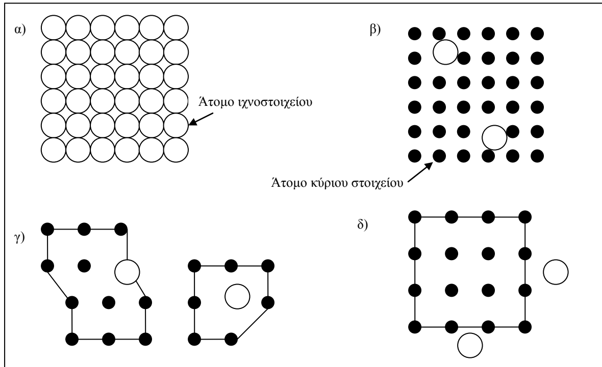
Εικόνα 3.3: Σχηματικό διάγραμμα των τεσσάρων τρόπων εμφάνισης ιχνοστοιχείων. (α) Ιχνοορυκτό, (β) Ιχνοστοιχείο σε καλά κρυσταλλωμένο ορυκτό, (γ) Ιχνοστοιχείο σε λεπτοκοκκώδες φτωγά κρυσταλλωμένο ορυκτό, (δ) Ιχνοστοιχείο προσροφημένο στην επιφάνεια ορυκτού. Πηγή: Rose et al., 1979 .
