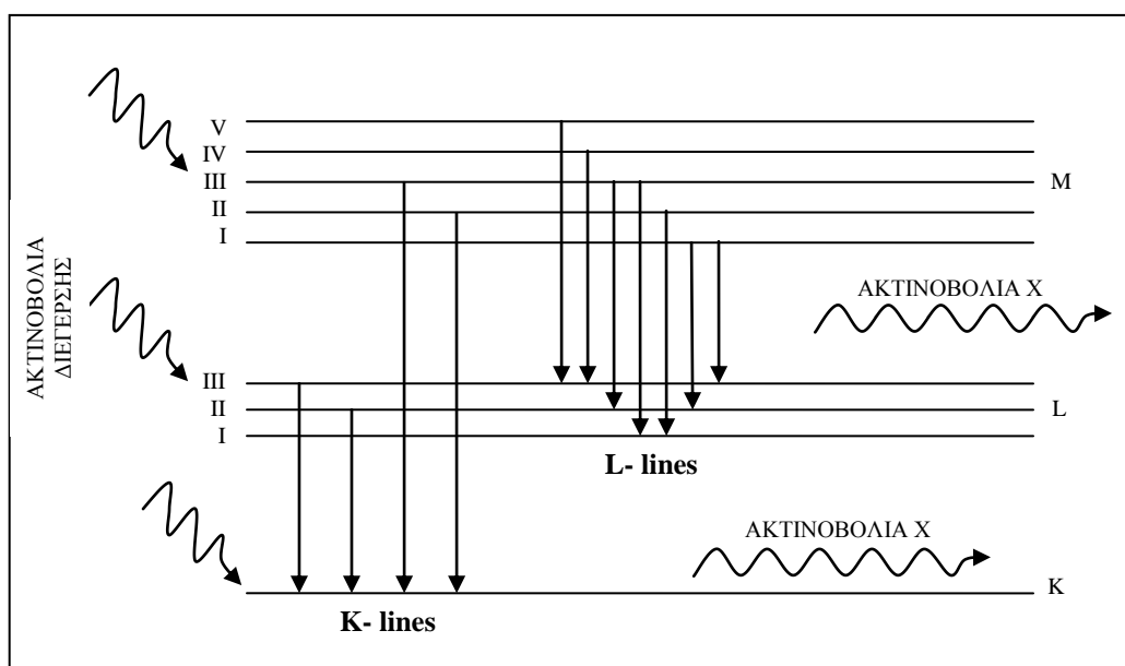
Εικόνα 4.2: Οι κύριες K και L XRF lines και οι αντίστοιχες μεταπτώσεις ηλεκτρονίων που τις προκαλούν.
