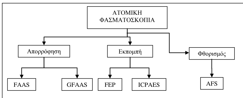
Εικόνα 3.2: Οι τεχνικές ατομικής φασματοσκοπίας.
