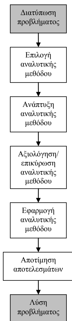
Σχήμα 1.4.: Συστηματική προσέγγιση στην επίλυση προβλημάτων αναλυτικής γεωχημείας.
