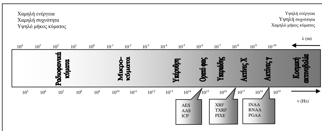
Εικόνα 3.1: Το ηλεκτρομαγνητικό φάσμα και σχετικές φασματοσκοπικές αναλυτικές τεχνικές.
