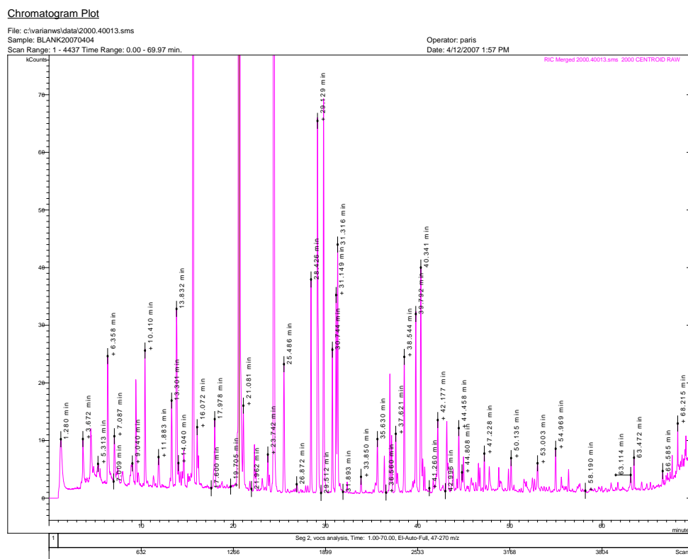
Εικόνα 5.6: Χρωματογράφημα GC-MS ενώσεων πηκτικών υδρογονανθράκων οι οποίες διαχωρίστηκαν από ένα δείγμα αεροζόλ. Σε κάθε κορυφή σημειώνεται ο χρόνος που απαιτήθηκε από μια συγκεκριμένη χημική ένωση για να διασχίσει το μήκος της χρωματογραφικής στήλης.
