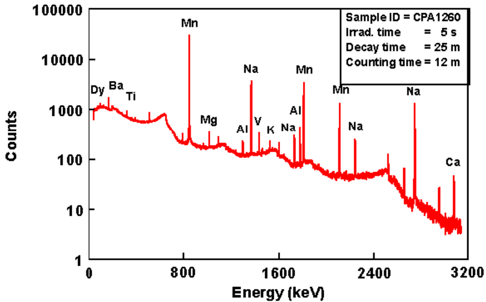
Εικόνα 4.9: Φάσμα ακτίνων γ δείγματος κεραμικού υλικού με χρόνους ενεργοποίησης 5', διάσπασης 25' και μέτρησης 12'. (Πηγή: http://en.wikipedia.org )
