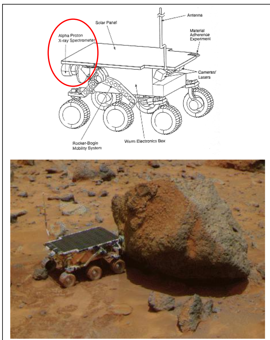
Εικόνα 4.1: Απεικόνιση του οχήματος Sojourner Rover διαστάσεων 65x48 cm και βάρους 10.6 kg στην επιφάνεια του πλανήτη Άρη, εξοπλισμένο με διάφορα είδη αισθητήρων και οργάνων για τη συλλογή δεδομένων από την επιφάνεια του πλανήτη. Μεταξύ αυτών και το APXS για τη χημική ανάλυση εδάφους και πετρωμάτων (Πηγή: NASA).
