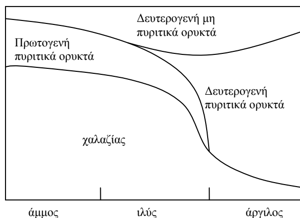
Εικόνα 2.9: Σχέση μεταξύ κοκκομετρίας και είδους ορυκτών σε εδάφη- ιζήματα.
