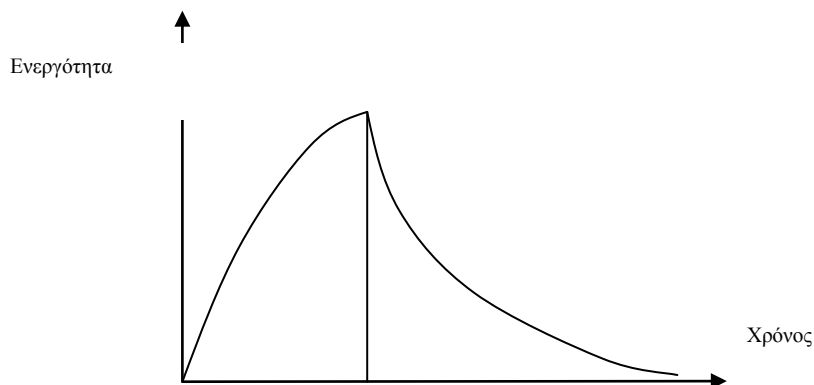
Εικόνα 4.6: Καμπύλες αύξησης και ελάττωσης της ραδιενέργειας ενός φυσικού δείγματος μετά από το βομβαρδισμό του με νετρόνια.
