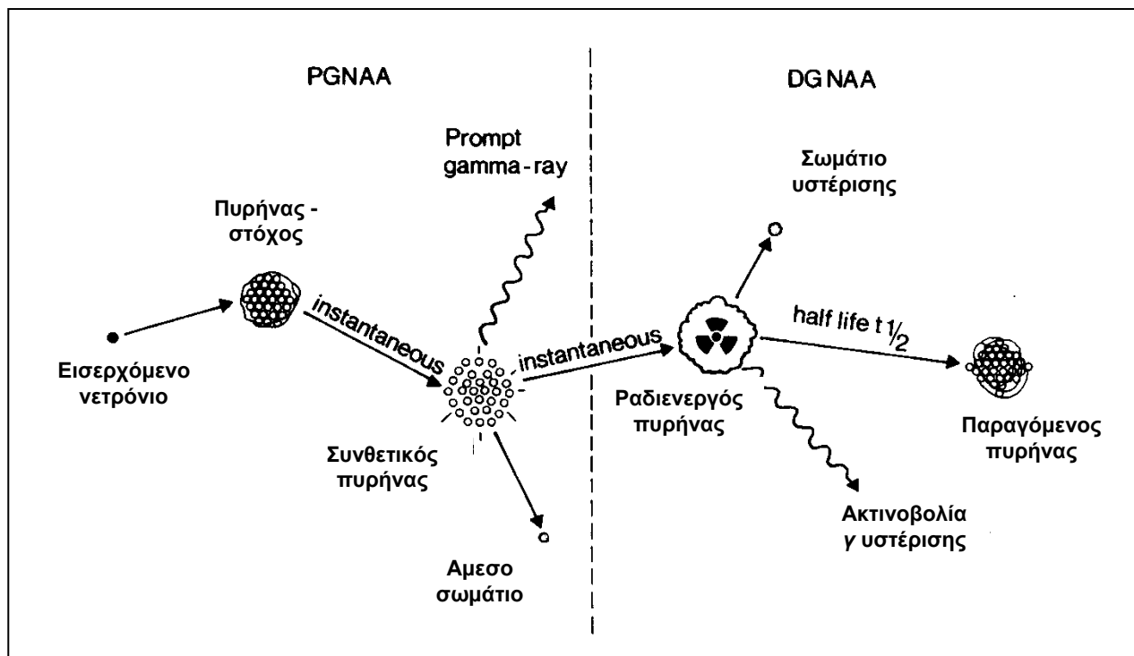
Εικόνα 4.7: Διαγραμματική αρχή λειτουργίας της αναλυτικής τεχνικής NAA. (Πηγή: http://en.wikipedia.org )
