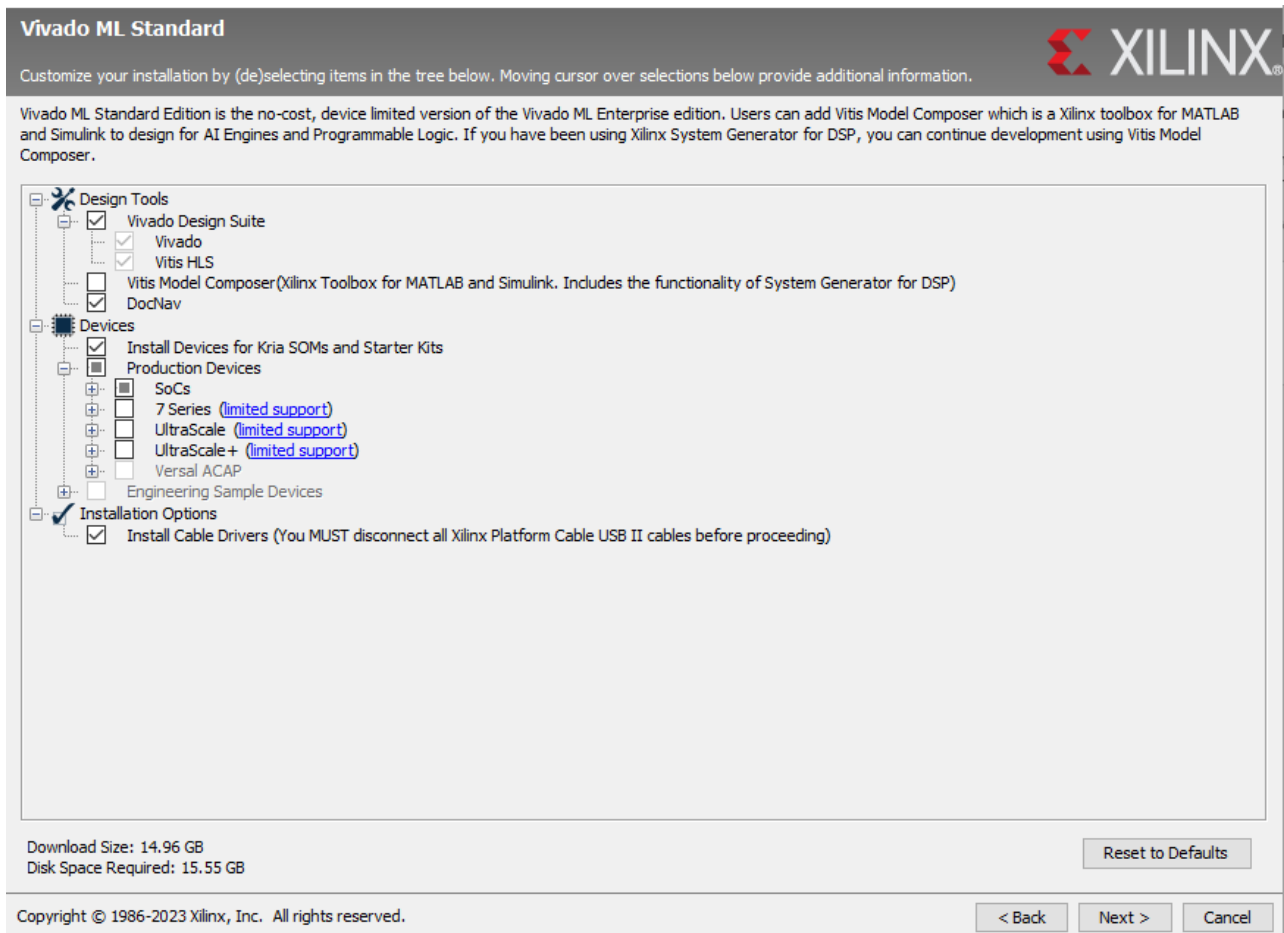
Εικόνα 15. Προσαρμοσμένη επιλογή στοιχείων Vivado
