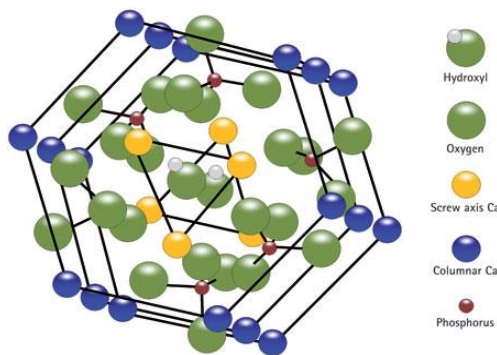
Μοριακή δομή του υδροξυαπατίτη
