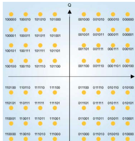
64-QAM
