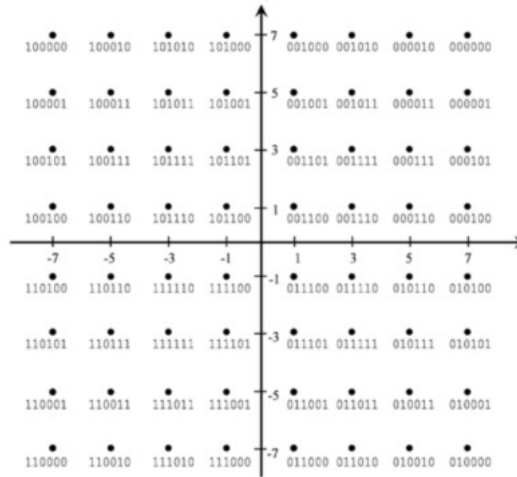
Συστήματα Ψηφιακής Ευρεκτομπής 64-QAM (6 bits/symbol)
