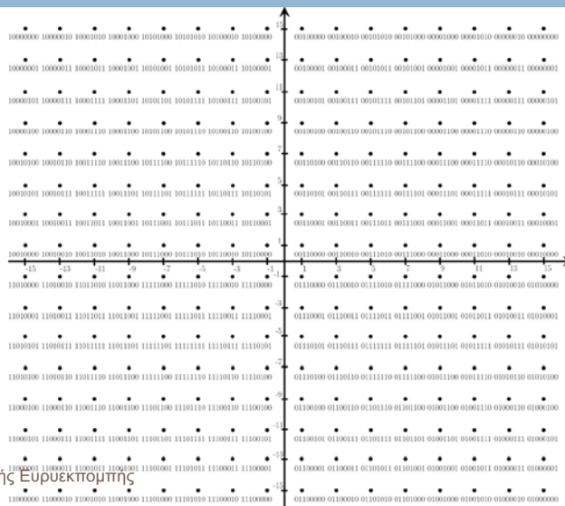
256-QAM (6 bits/symbol) μόνο στο DVB-T2
