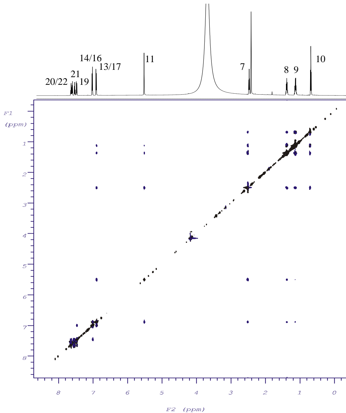
(αριστερά) Πείραμα ROESY του EXP-3174 σε DMSO. (δεξιά) Σε μεγέθυνση η αρωματική περιοχή.
