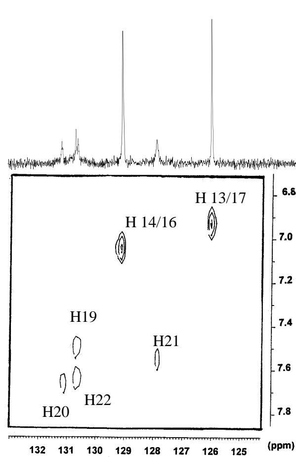
(αριστερά) Ετεροπυρηνικό πείραμα 2D ^{13}\text{C} - ^1\text{H} του EXP-3174 σε DMSO. (δεξιά) Αρωματική περιοχή.
