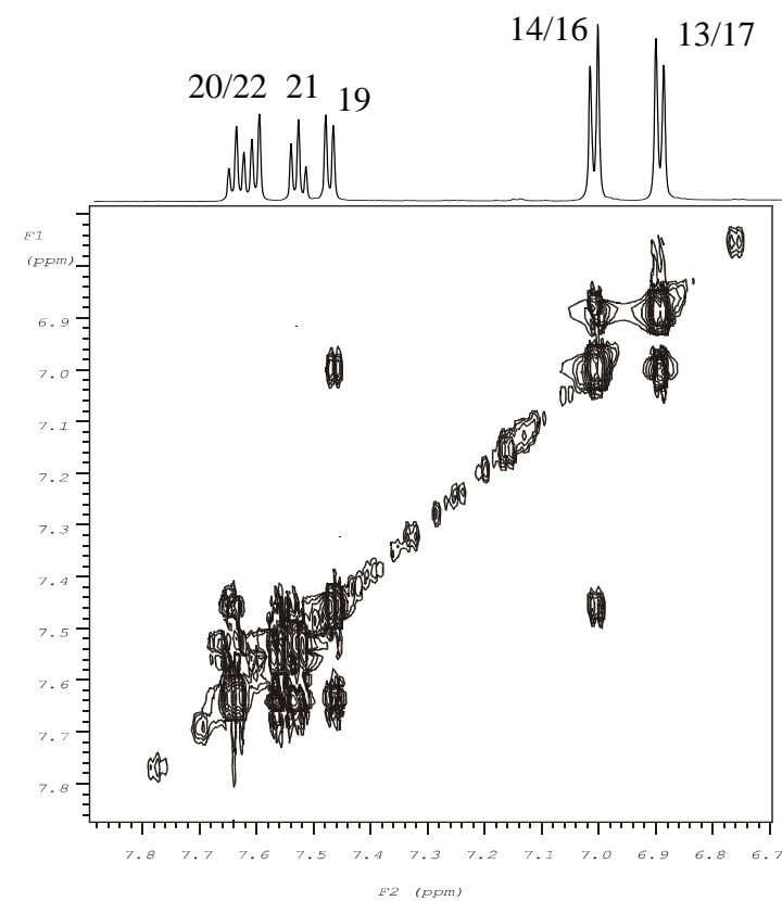
(αριστερά) Πείραμα ROESY του EXP-3174 σε DMSO. (δεξιά) Σε μεγέθυνση η αρωματική περιοχή.
