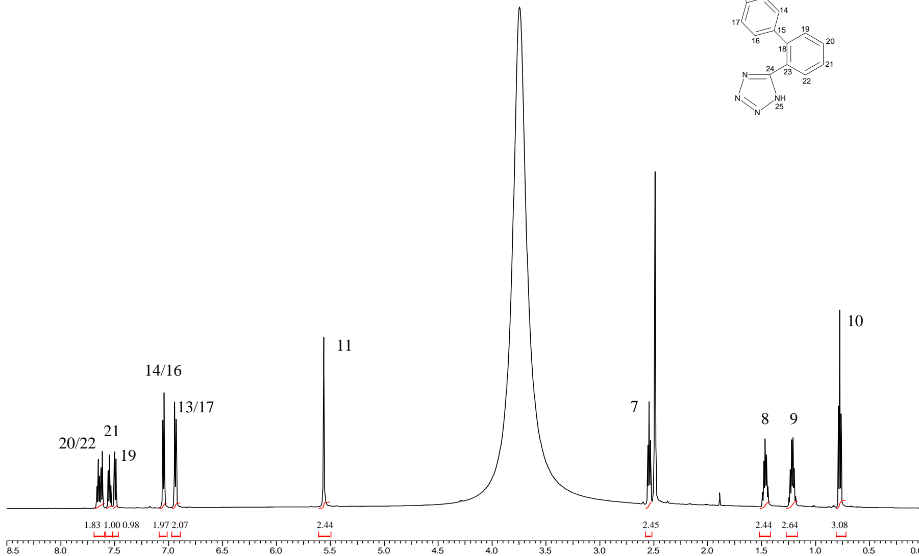
Φάσμα πρωτονίου του EXP-3174 σε DMSO.
