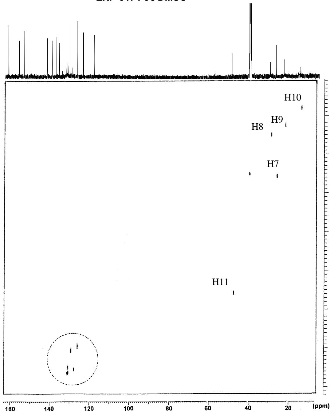
(αριστερά) Ετεροπυρηνικό πείραμα 2D ^{13}\text{C} - ^1\text{H} του EXP-3174 σε DMSO. (δεξιά) Αρωματική περιοχή.
