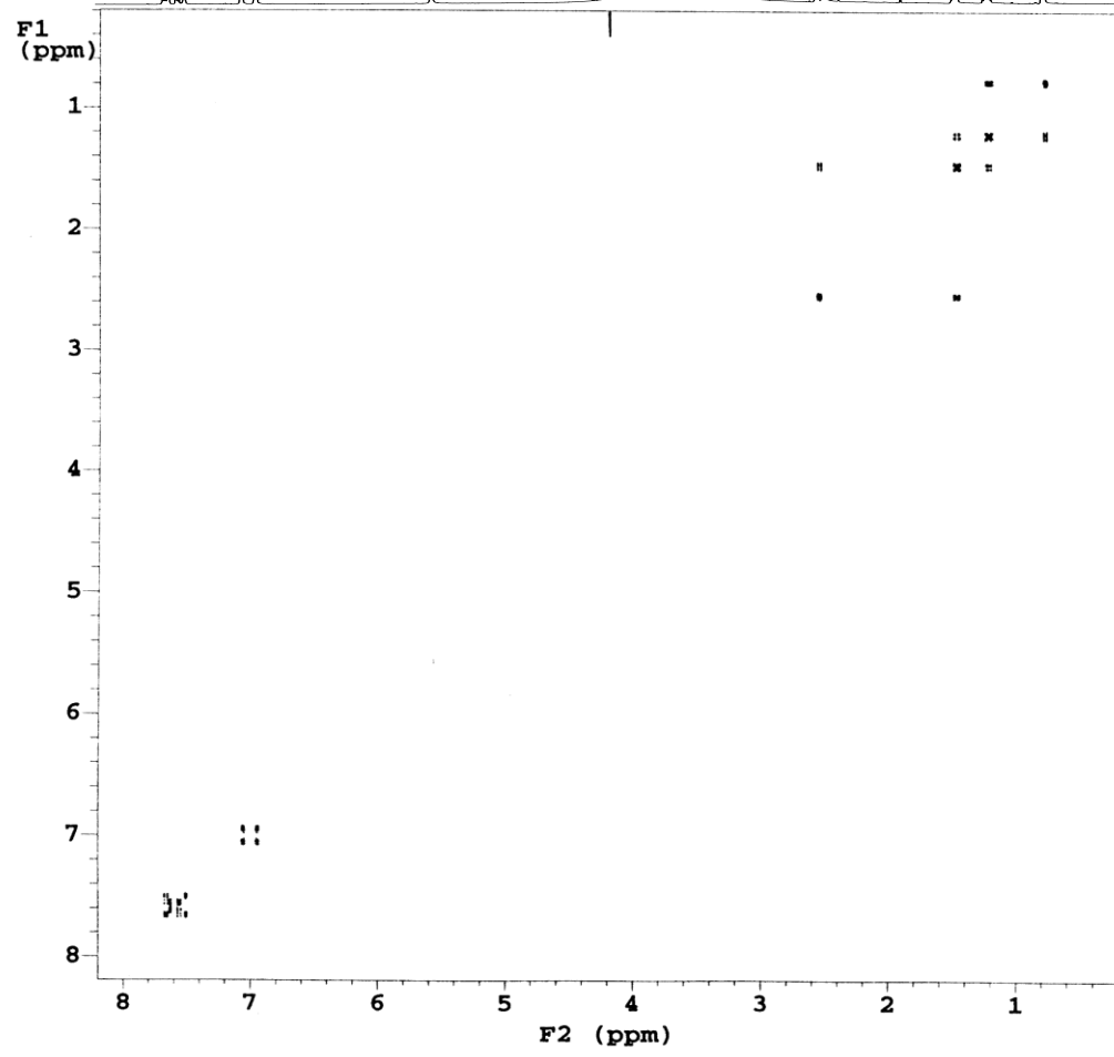
(αριστερά) Πείραμα DQF-COSY του EXP-3174 σε DMSO. (δεξιά) Αρωματική περιοχή.
