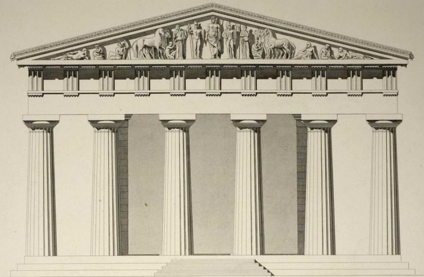
ANSICHT DER OESTLICHEN GIEBELSEITE
