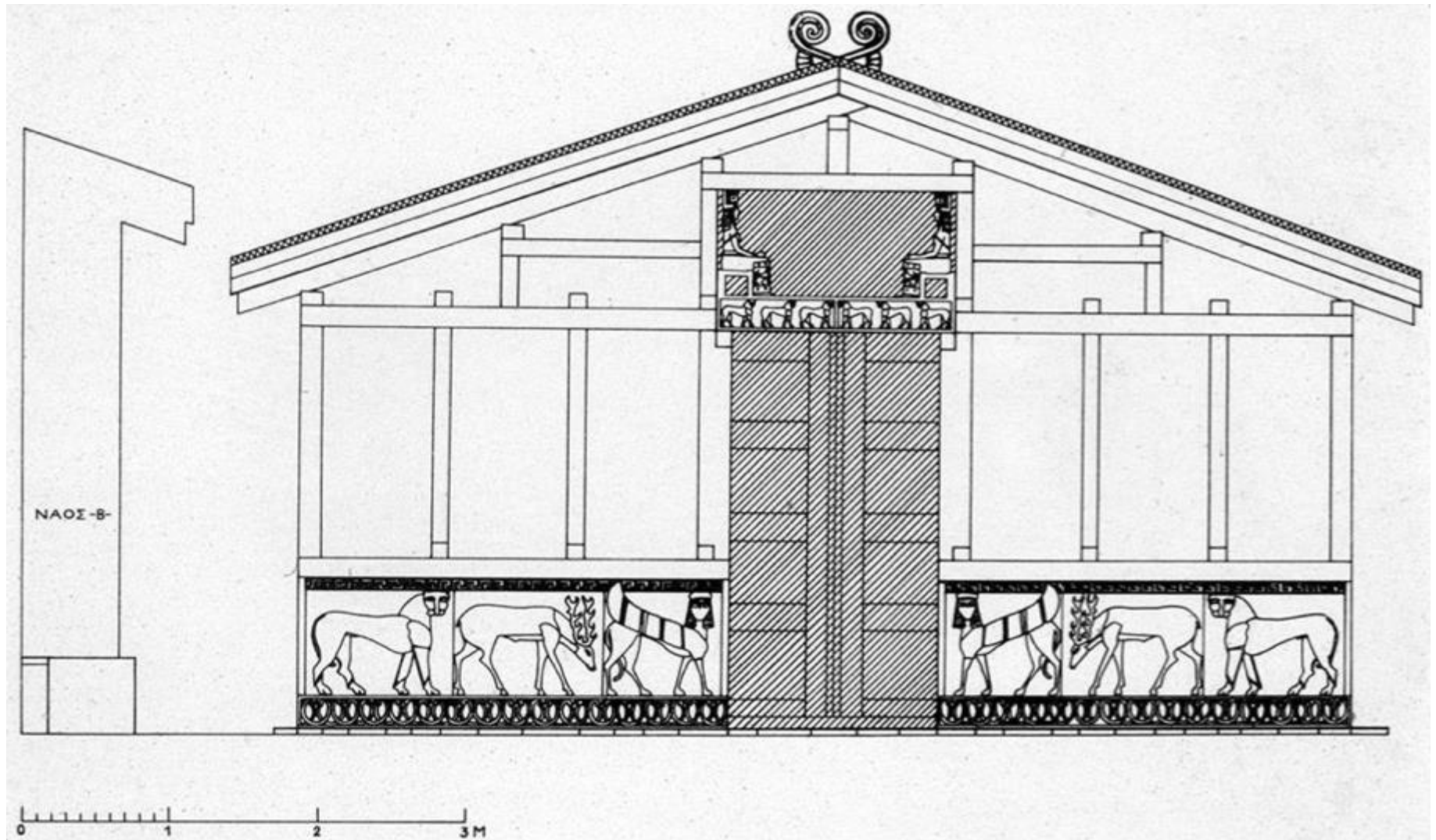
σχεδιαστική αναπαράσταση της πρόσοψης του ναού Α του Πρινιά
