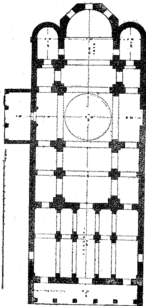
Σχέδιον τοῦ Ναοῦ Παναγίας τῆς «Χρυσοκεφάλου»
