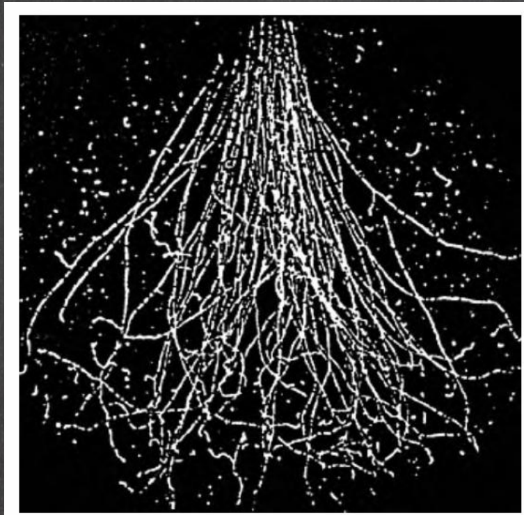
e^- 9.3 MeV σε σε θάλαμο φυσαλίδων προπανίου
