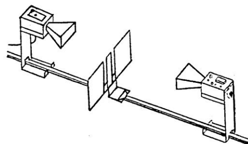
Εικόνα 13. Στήσιμο εξοπλισμού διπλής σχισμής.
