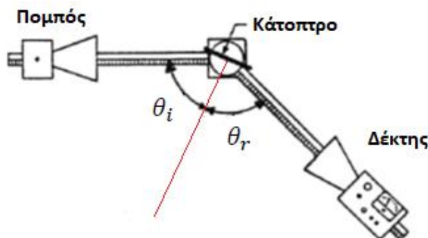
Εικόνα 6. Γωνίες προσπτώσεως, \theta_i , και ανακλάσεως, \theta_r .
