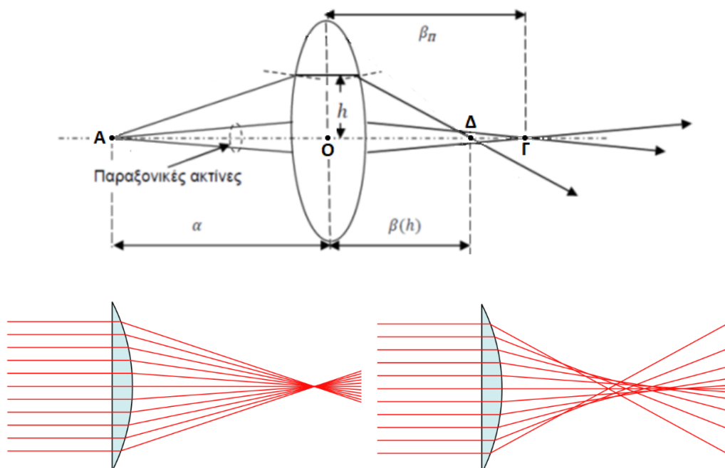
Σχήμα 1. Επίδραση της σφαιρικής εκτροπής στην εστιακή απόσταση φακού. Άνω: Η πορεία των κοντινών στον κύριο άξονα, παραξονικών, ακτίνων, οι οποίες εστιάζονται κατά προσέγγιση στην εστία, Γ, καθώς και των μακρινότερων ακτίνων, των οποίων η εστίαση εξαρτάται από το ύψος από το Ο, h . Κάτω αριστερά: ένας τέλειος φακός, χωρίς σφαιρική εκτροπή, όπου όλες οι ακτίνες μαζεύονται στην εστία. Κάτω δεξιά: ένας πραγματικός φακός, με σφαιρική εκτροπή: Διαφορετικές ακτίνες τέμνουν τον κύριο άξονα σε διαφορετικό σημείο, μάλιστα, όσο πιο μακριά βρίσκονται οι ακτίνες από τον κύριο άξονα, τόσο πιο κοντά στο φακό τον τέμνουν. (θετική σφαιρική εκτροπή).
