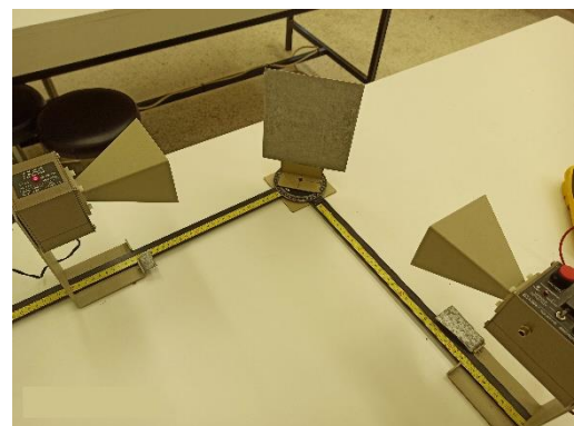
Εικόνα 7. Παράδειγμα, \theta_r = \theta_i \approx 45^\circ .
