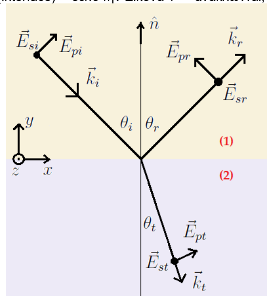
Εικόνα 1. Γωνίες, συνιστώσες ηλεκτρικού πεδίου και κυμαανύσματα σε διεπιφάνεια [4].
