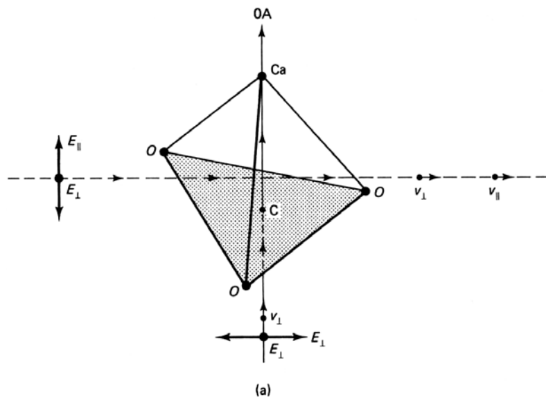
Ασβεστίτης \text{CaCO}_3
