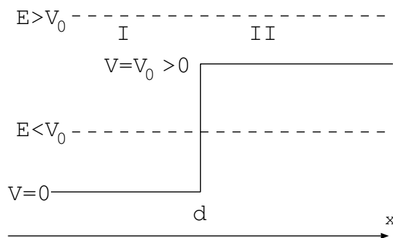
Σχήμα 4: Βήμα δυναμικού με V_0 > 0 .
