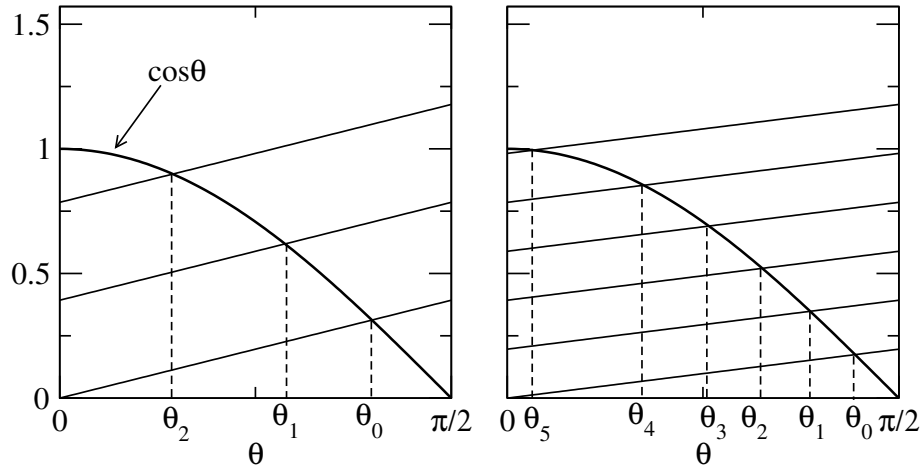
Σχήμα 2: Γραφική λύση της εξ. (129) για \lambda = \frac{\sqrt{2m|V_0|}}{\hbar}d = 4 (αριστερά) και \lambda = 8 (δεξιά). Τα σημεία τομής των ευθειών με την καμπύλη \cos \theta αντιστοιχούν στις λύσεις \theta_n στον άξονα των \theta .
