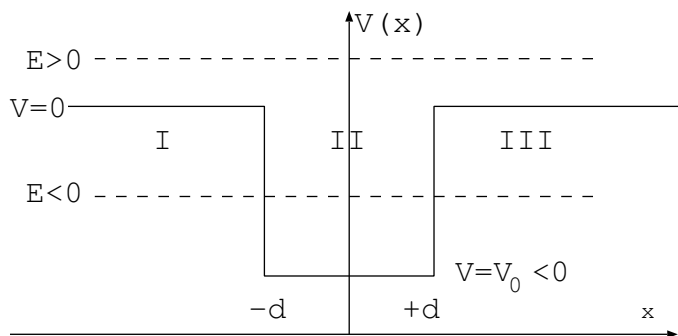
Σχήμα 1: Πηγάδι δυναμικού σε μία διάσταση.
