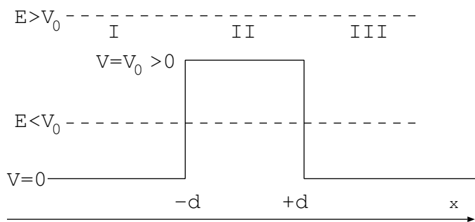
Σχήμα 3: Φραγμός δυναμικού σε μία διάσταση.
