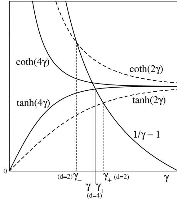
Σχήμα 5: Γραφική λύση των εξ. (172) για d = 2 και d = 4 .
