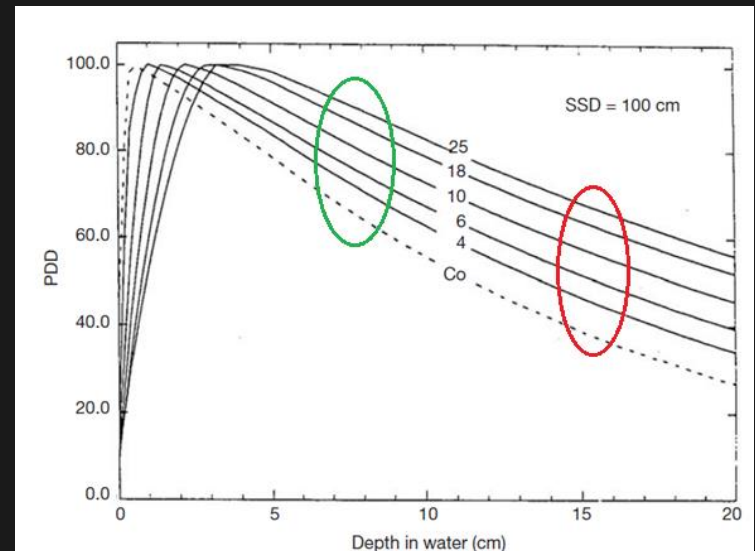
photons
