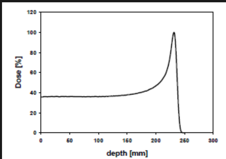
protons
