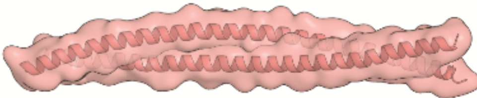
Σπειροειδής έλικα δύο αλυσίδων
