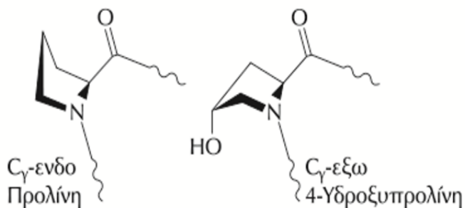
EIKONA 1 Η C \gamma -ενδο διαμόρφωση της προλίνης και η C \gamma -εξω διαμόρφωση της 4-υδροξυπρολίνης.
