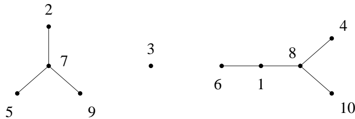
Σχήμα 5.1: Ένα δάσος με τρεις συνιστώσες στο σύνολο κορυφών [10].
