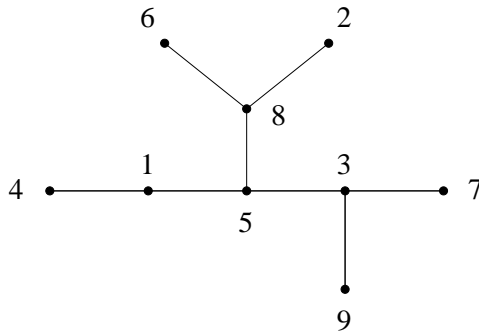
Σχήμα 4.6: Ένα δένδρο στο σύνολο κορυφών [9].
