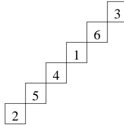
Σχήμα 3.14: Ένα λοξό ταμπλώ με λέξη γραμμών (2, 5, 4, 1, 6, 3) .
