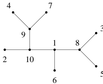
Σχήμα 5.4: Ένα εναλλασσόμενο δένδρο με 10 κορυφές.
