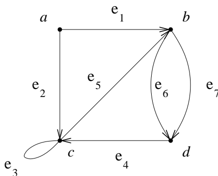
Σχήμα 4.1: Ένα κατευθυνόμενο γράφημα.
