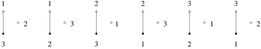
Σχήμα 4.9: Τα δάση στο σύνολο κορυφών \{1, 2, 3\} με δύο ρίζες.
