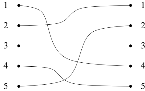
Σχήμα 2.1: Αντιστροφές της μετάθεσης (4, 1, 3, 5, 2) .
