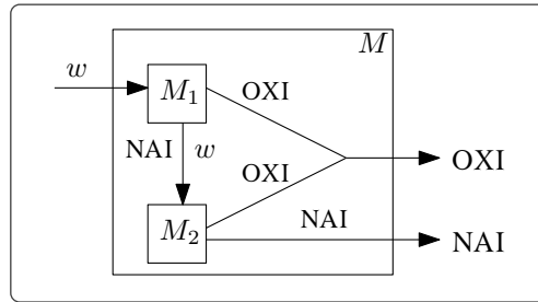
Σχήμα 1.5.1: Η ΤΜ M που αποφασίζει (ημι-αποφασίζει) την L_1 \cap L_2 .
