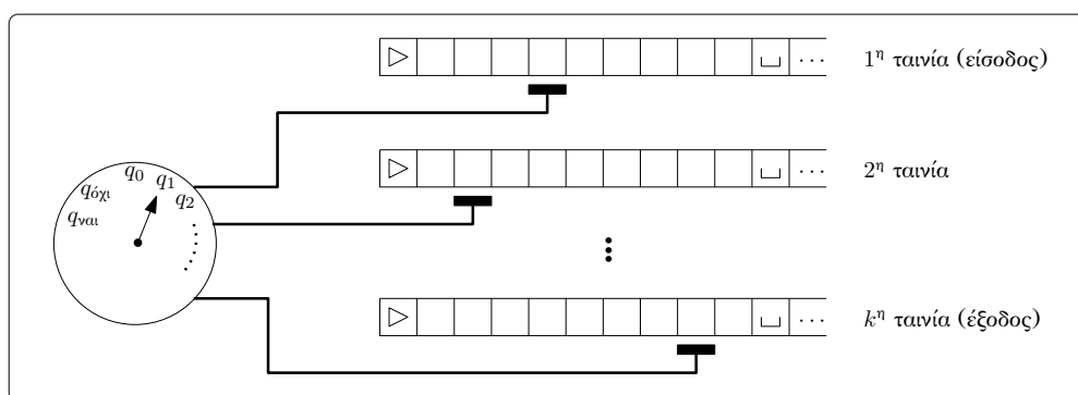
Σχήμα 1.3.1: Σχηματική αναπαράσταση μίας TM k -ταινιών.
