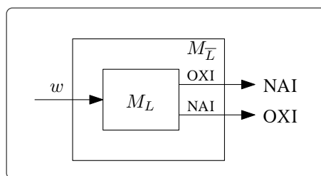
Σχήμα 1.5.4: Η ΤΜ M_{\bar{L}} που αποφασίζει την \bar{L} .
