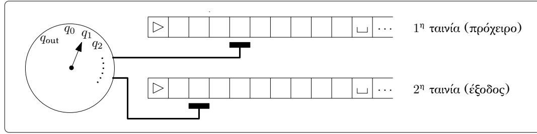
Σχήμα 1.2.17: Σχηματική αναπαράσταση ενός απαριθμητή.
