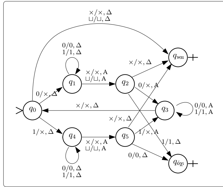
Σχήμα 1.2.12: Η ΤΜ του Παραδείγματος 1.2.33.
