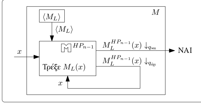
Σχήμα 8.4.2: Η OTM M στην απόδειξη του Θεωρήματος 8.4.4.
