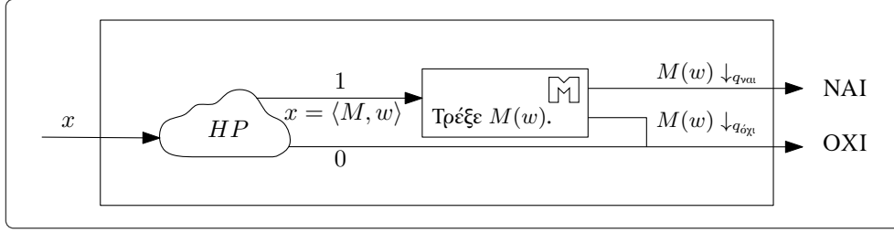
Σχήμα 8.1.2: Η OTM που αποφασίζει την L_{\text{Αποδοχής}} .
