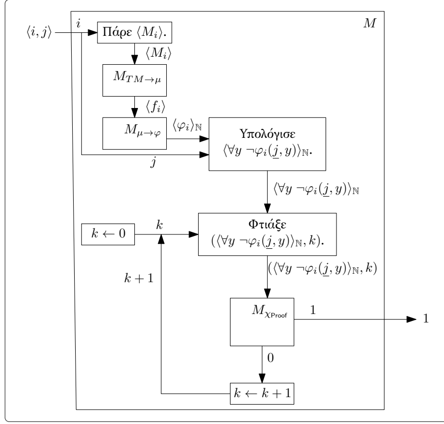
Σχήμα 7.3.2: Η ΤΜ M που υπολογίζει τη συνάρτηση g στην απόδειξη του Θεωρήματος 7.3.7 (με \langle \varphi_i \rangle_{\mathbb{N}} συμβολίζουμε τον αριθμό Gödel της πρόταση \varphi_i , δες Παράγραφο Α.5.1).
