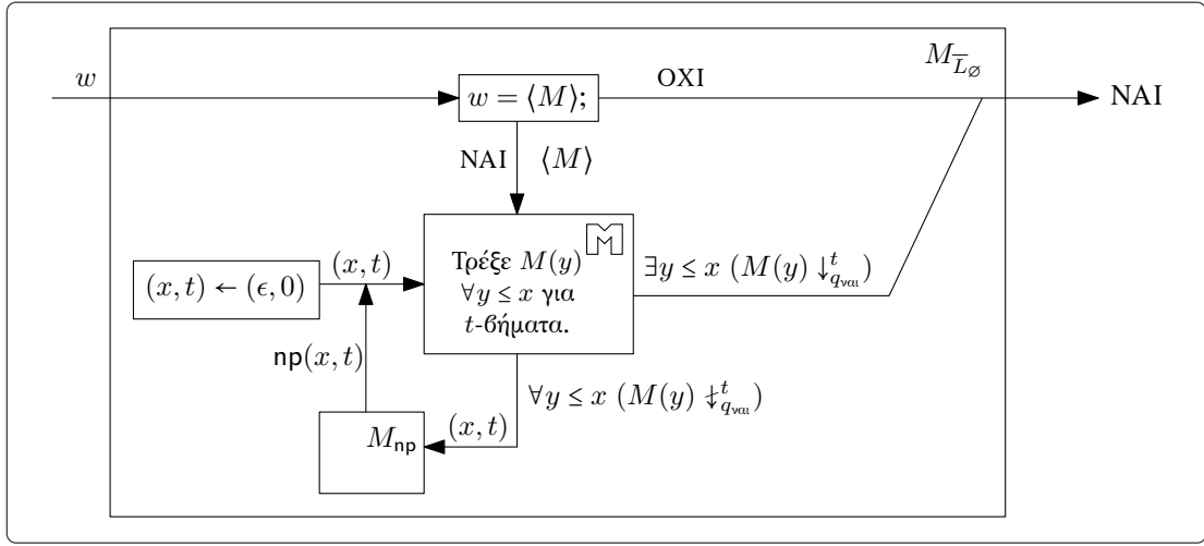
Σχήμα 8.3.1: Η ΤΜ που ημι-αποφασίζει την \bar{L}_\emptyset , όπου M_{np} η ΤΜ της Παρατήρησης 1.4.19.
