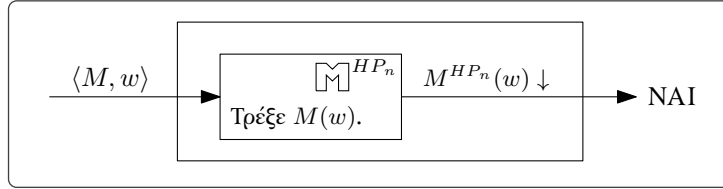
Σχήμα 8.2.3: Η OTM στην απόδειξη του Λήμματος 8.2.7.
