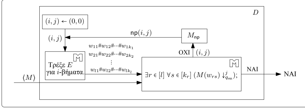
Σχήμα 6.2.6: Η ΤΜ D στην απόδειξη του Θεωρήματος 6.2.2.
