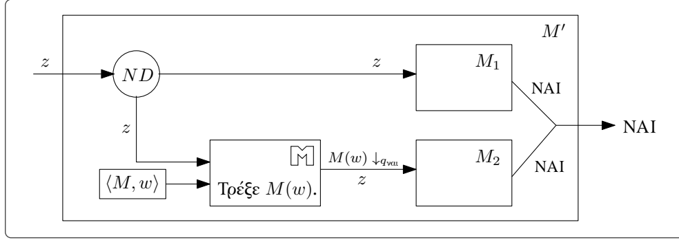
Σχήμα 6.2.2: Η ΤΜ M' στην απόδειξη του ότι L_P \in RE \Rightarrow \textcircled{1} στο Θεώρημα 6.2.2.
