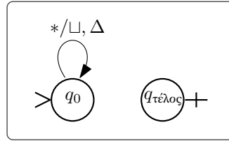
Σχήμα 1.2.3: Το διάγραμμα καταστάσεων της TM του Παραδείγματος 1.2.21 (το σύμβολο * παίρνει όλες τις τιμές του \Sigma \setminus \{\triangleright\} ).
