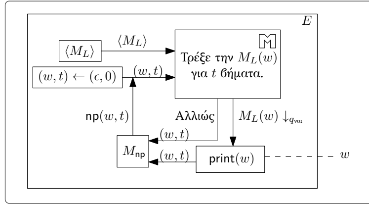
Σχήμα 1.4.3: Ο απαριθμητής E που απαριθμεί την L όταν η ΤΜ M_L την ημι-αποφασίζει. Γράφουμε \text{print}(w) αντί για το «Σθήσε τη δεύτερη ταινία γράψε w και πήγαινε q_{\text{out}} » που είχαμε γράψει στον απαριθμητή του Σχήματος 1.2.21.
