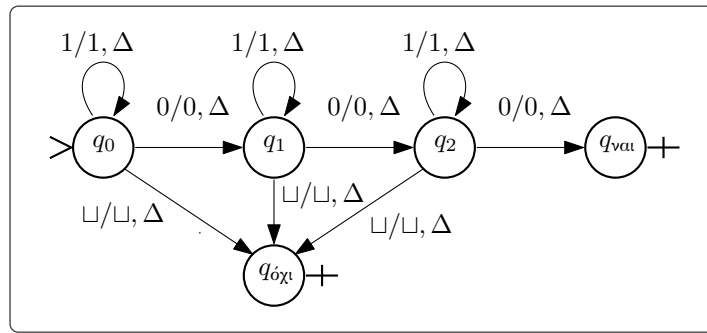
Σχήμα 1.2.II: Η TM του Παραδείγματος 1.2.32.
