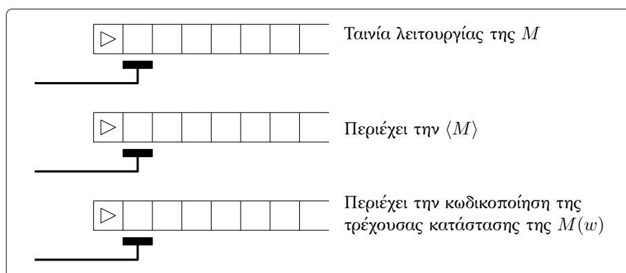
Σχήμα 1.4.1: Οι τρεις ταινίες μίας Καθολικής TM (με είσοδο \langle M, w \rangle ).
