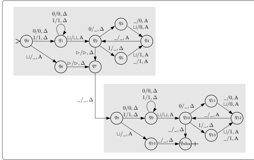
Σχήμα 1.2.6: Η TM που υπολογίζει τη συνάρτηση του Παραδείγματος 1.2.10.
