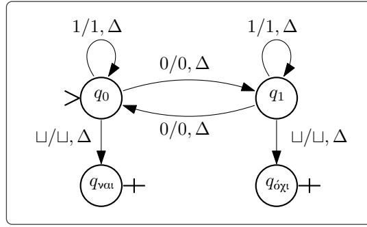
Σχήμα 1.2.10: Η ΤΜ του Παραδείγματος 1.2.31.
