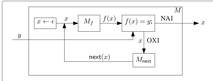
Σχήμα 1.2.14: Η ΤΜ που υπολογίζει τη συνάρτηση f^{-1} .
