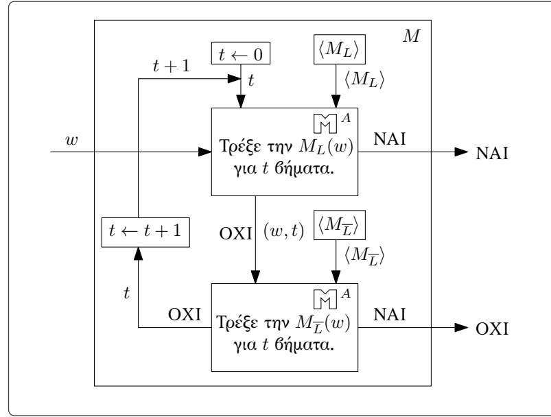
Σχήμα 8.1.5: Η ΤΜ M που αποφασίζει την L όταν L \in \text{RE}^A \cap \text{co-RE}^A (ο λόγος που χρησιμοποιούμε τον συμβολισμό \mathbb{M}^A αναφέρεται στην Υποσημείωση 1 στη Σελίδα 171).
