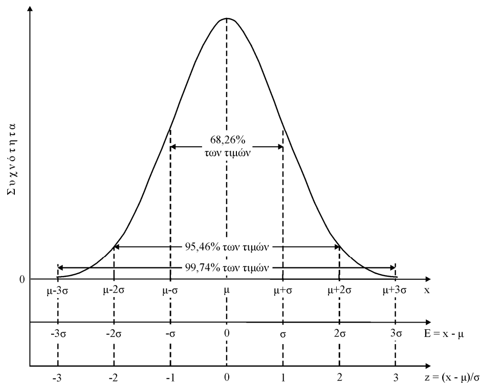
Σχήμα 2-4. Τυπική καμπύλη κανονικής κατανομής (καμπύλη Gauss) και διάφορα χαρακτηριστικά σημεία της.
