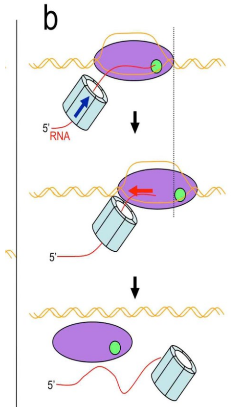
(β) Ο Rho μετακινείται κατά μήκος του νεοσυντιθέμενου RNA ως το σύμπλοκο επιμήκυνσης όπου «σπρώχνει» το RNA έξω από το σύμπλοκο επιμήκυνσης.
