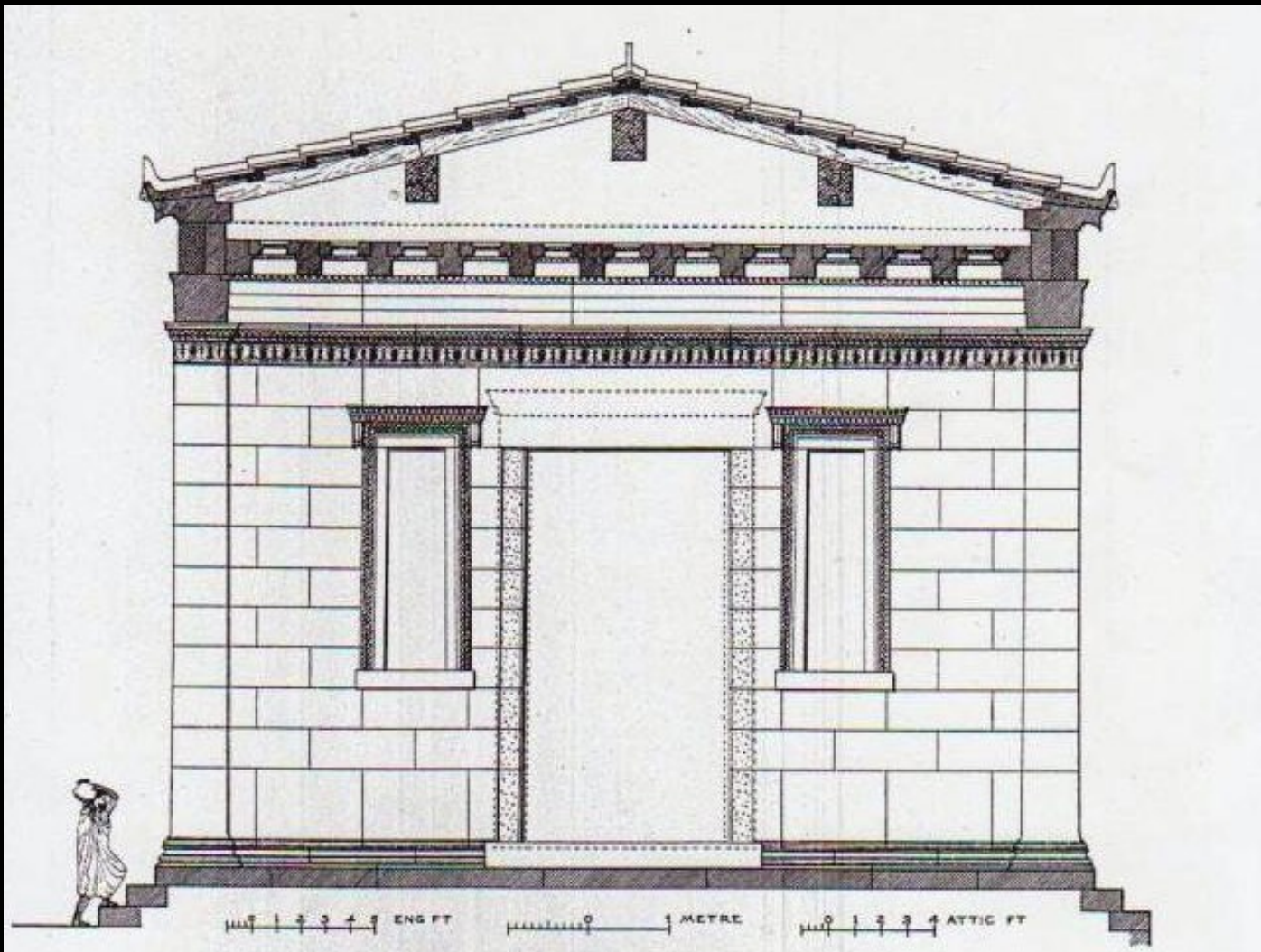
Ο ανατολικός τοίχος του ναού χωρίς την πρόσταση.
