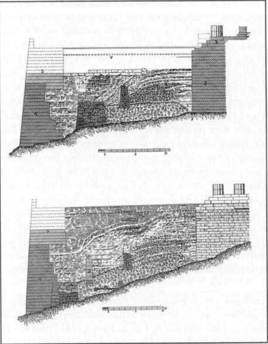
Εικ. 1 Στρωματογραφικές τομές νότια του Παρθενώνος (Dörpfeld)
