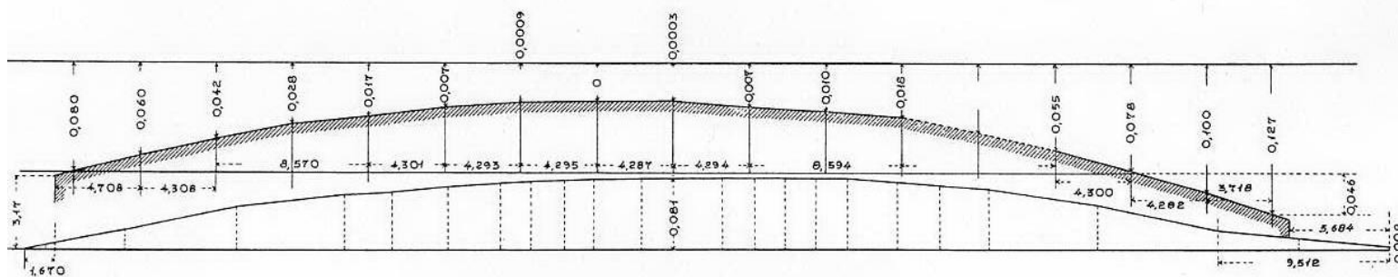
44. Καμπυλότητες τῶν στρώσεων 6, 7 καὶ 8 (κατὰ Σῖνον).
