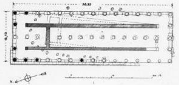
DER TEMPEL DES APOLLON ZU THERMOPYLAE 1. DER GRUNDRISS 2. DAS GEDÄULDE, VON G. SAWERHALD RECONSTRUIERT
