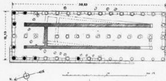
DER TEMPEL DES APOLLON ZU THERMOPYLAE
