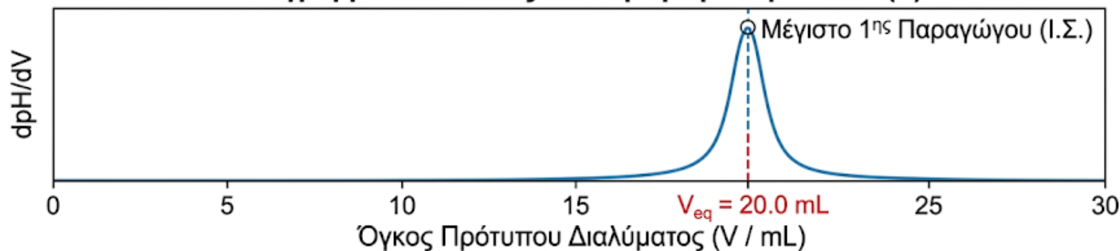
Διάγραμμα 2: Μέθοδος 1 ης Παραγώγου d\text{pH}/dV = f(V)
