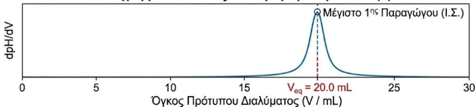
Διάγραμμα 2: Μέθοδος 1ης Παραγώγου \text{dpH}/\text{dV} = f(V)
