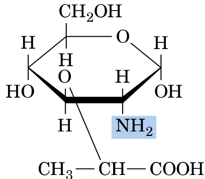
Μουραμικό οξύ
