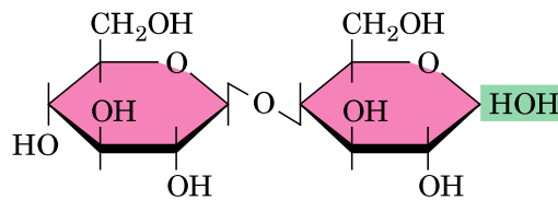
Κελλοβιόζη (γλυκόζη-β-1,4-γλυκόζη)
