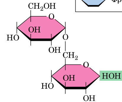
Ισομαλτόζη (γλυκόζη-α-1,6-γλυκόζη)
