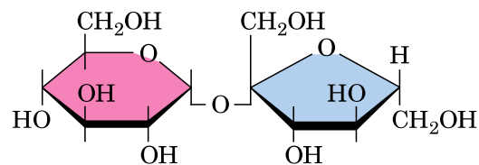
Σακχαρόζη (γλυκόζη-1α-β2-φρουκτόζη)
