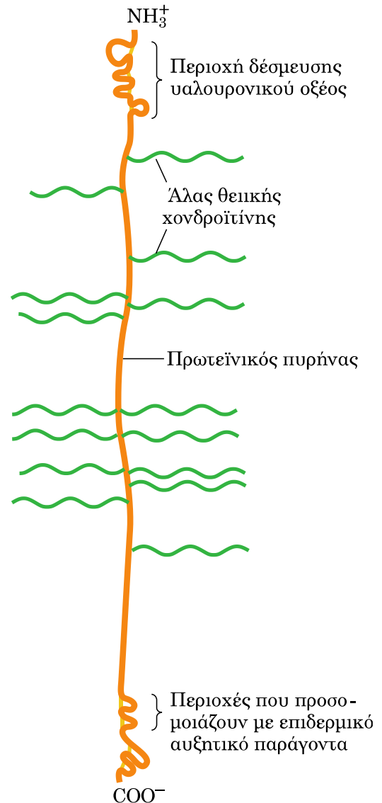
(α) Βερσικάνη
