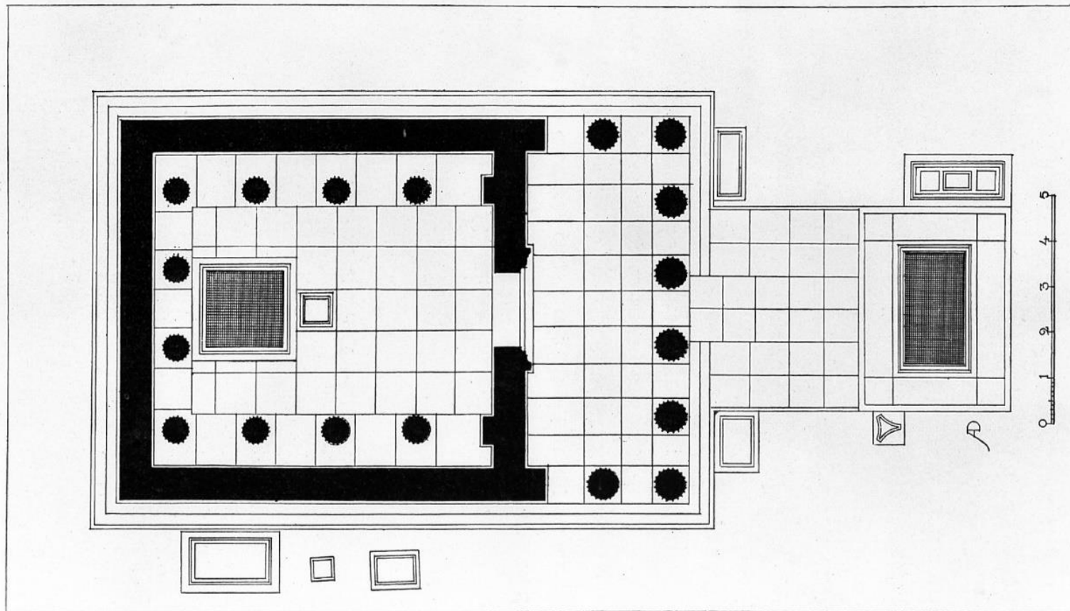
PLAN RESTAURÉ DU TEMPLE D'ARTÉMIS.
