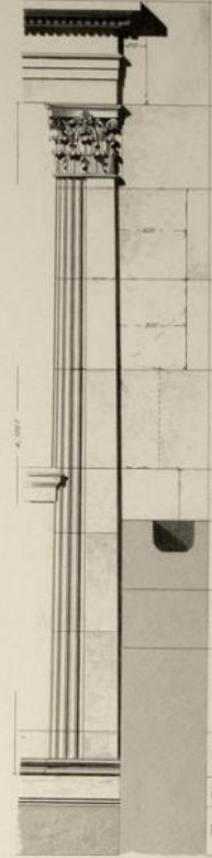
3 AUFRIß D. N. ECKE
