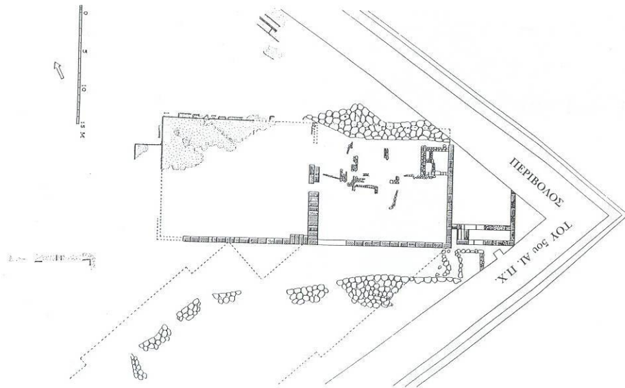
114. Κάτοψη του ιερού του Πανδίωνος (κατά G. Ph. Stevens).
