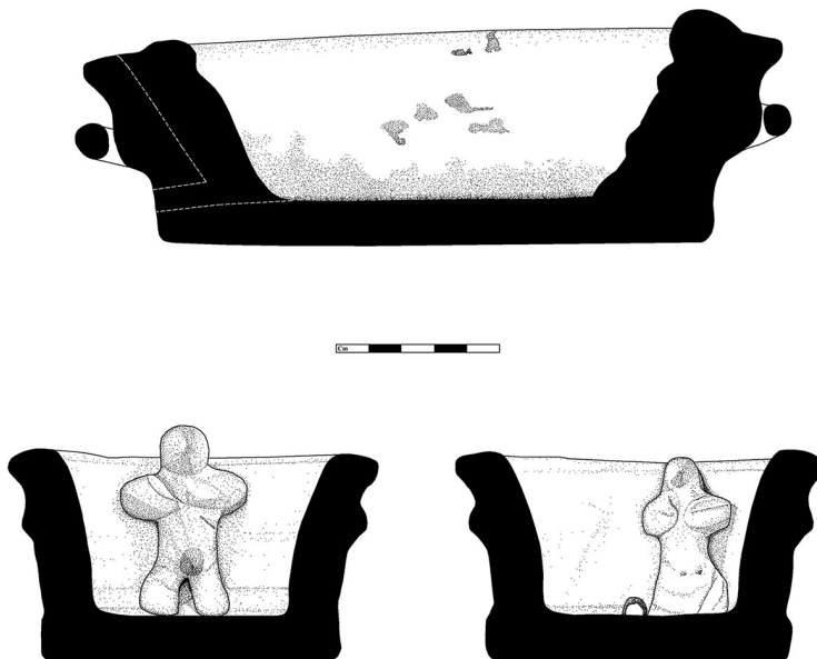
Εικ. 2. Κατά μήκος και εγκάρσιες σχεδιαστικές τομές του αντικειμένου (σχεδίαση Ντίνα Βασιλοπούλου).
