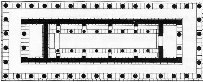
39. Κάτοψη αρχαϊκού Ηραϊού Ολυμπίας. Γύρω στο 600 π.Χ.
