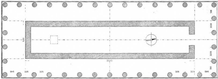
39. Κάτοψη αρχαϊκού Ηραϊού Ολυμπίας. Γύρω στο 600 π.Χ.
